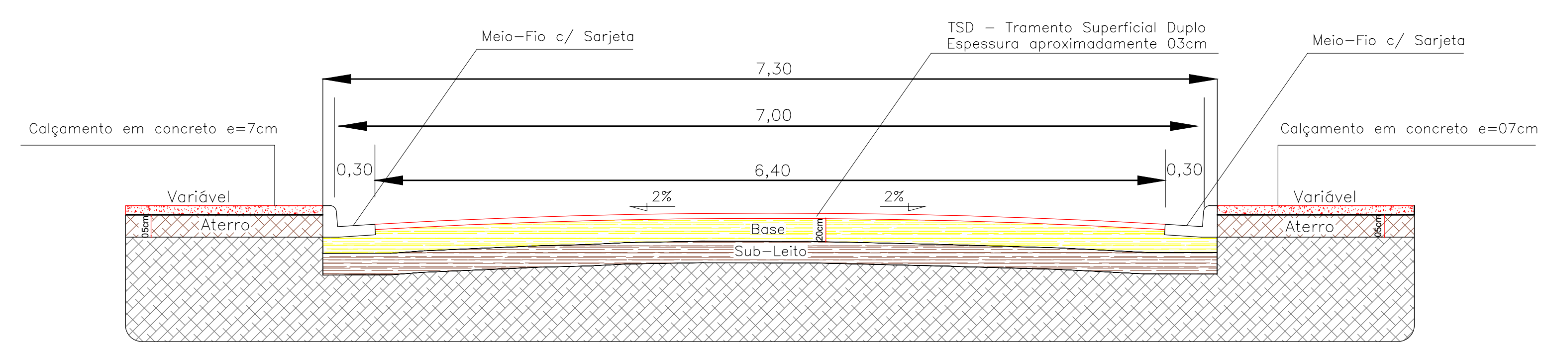
PERFIL TRANSVERSAL - PISTA 7,00m. SEM ESCALA
