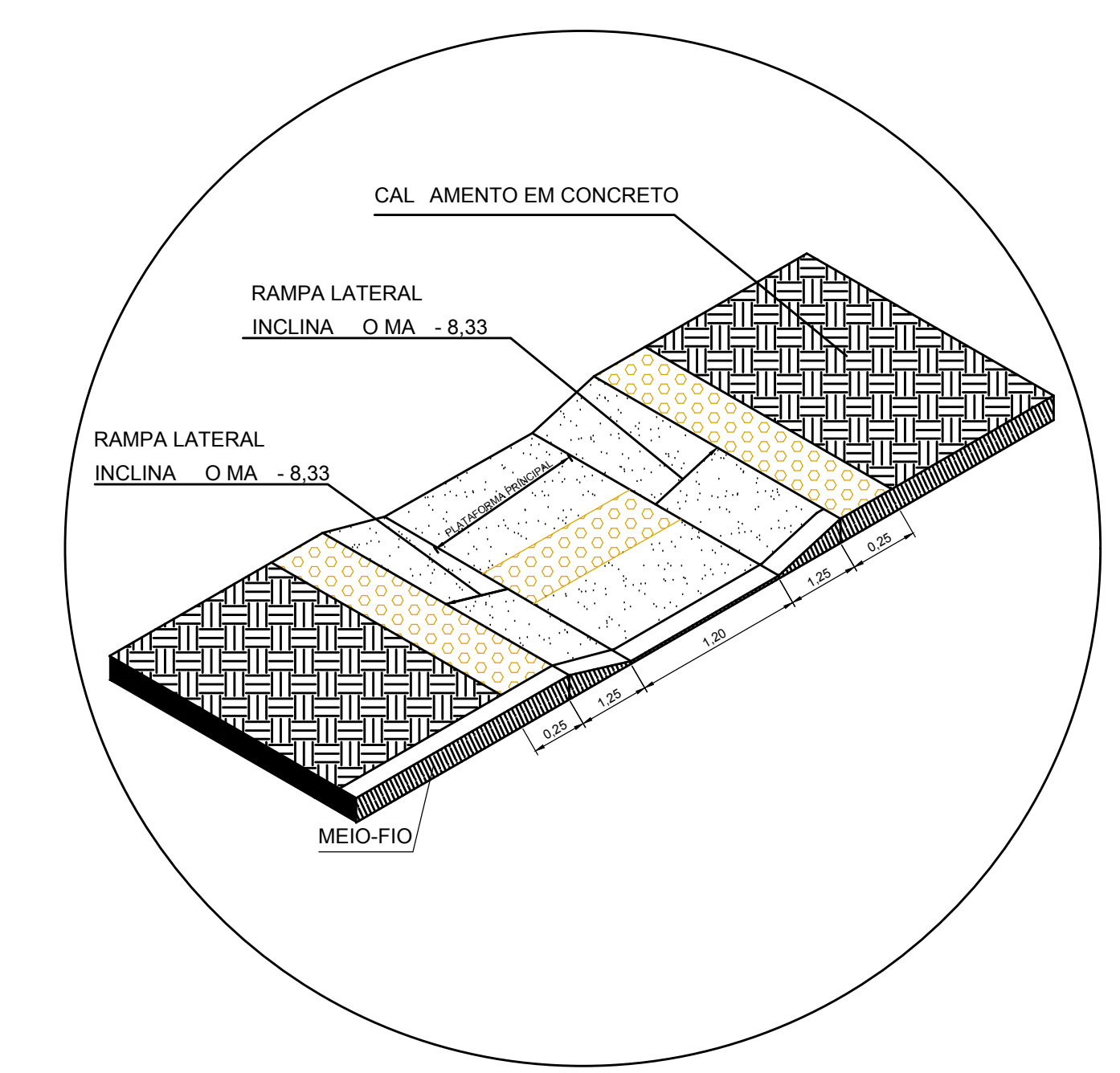
DETALHE DE RAMPA DE ACESSIBILIDADE sem escala
