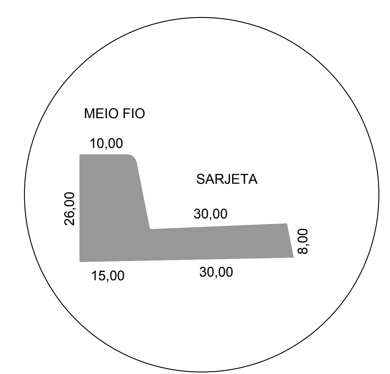
DETALHE MEIO FIO C/ SARJETA sem escala
