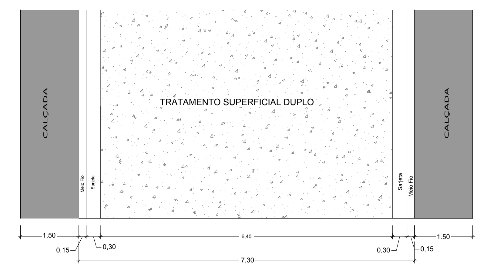
DETALHE DE VIAS SEM ESCALA
