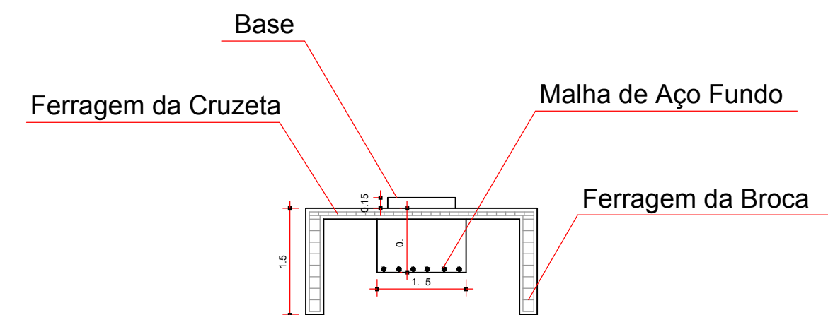
DETALHE - BASE RESERVATÓRIO SEM ESCALA
