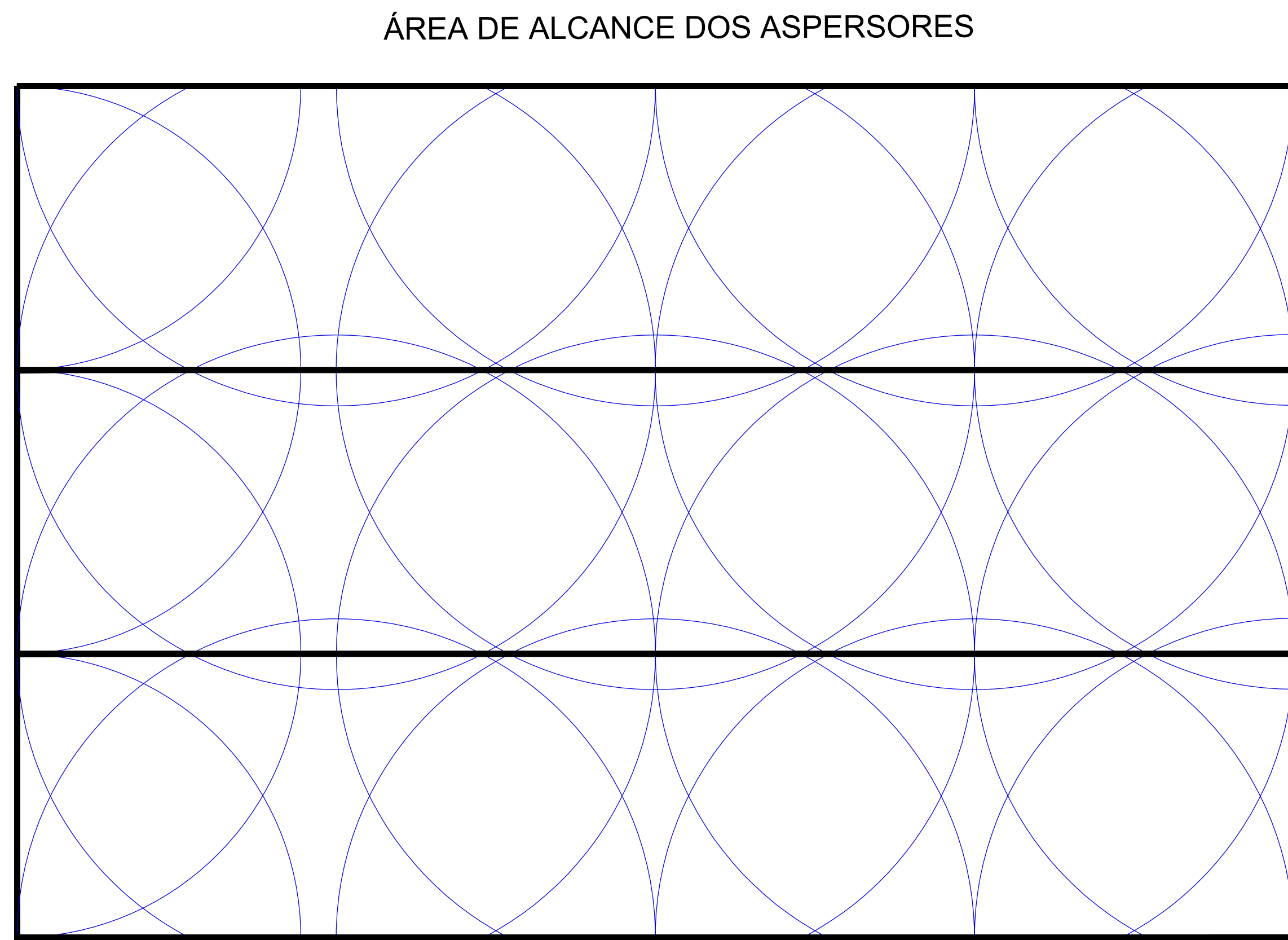
PLANTA DE IRRIGAÇÃO ESCALA 1:100
