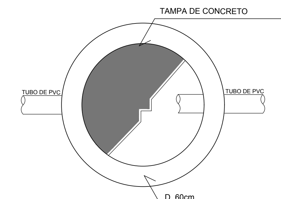
PLANTA BAI A - CAI A DE PASSAGEM SEM ESCALA
