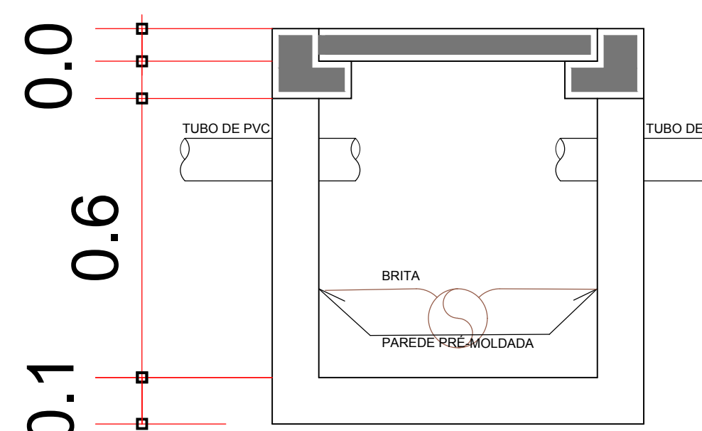
CORTE - CAI A DE PASSAGEM SEM ESCALA
