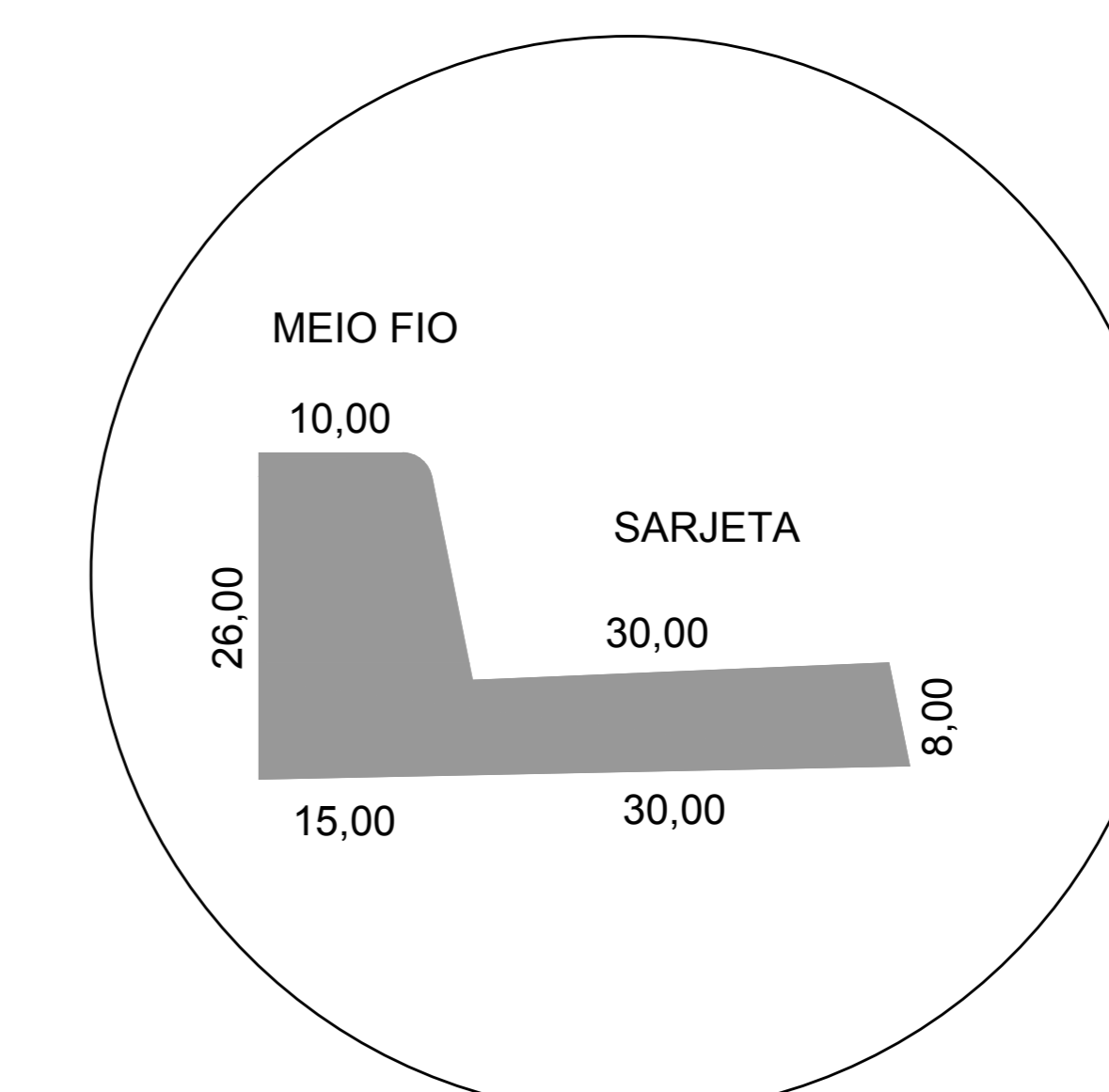
DETALHE MEIO FIO C/ SARJETA
