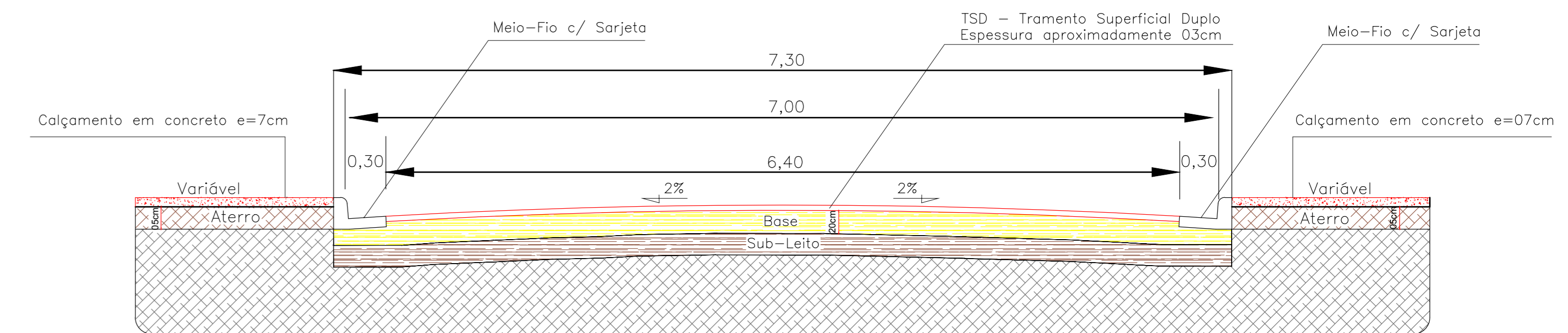
PERFIL TRANSVERSAL - PISTA 7,00m.
