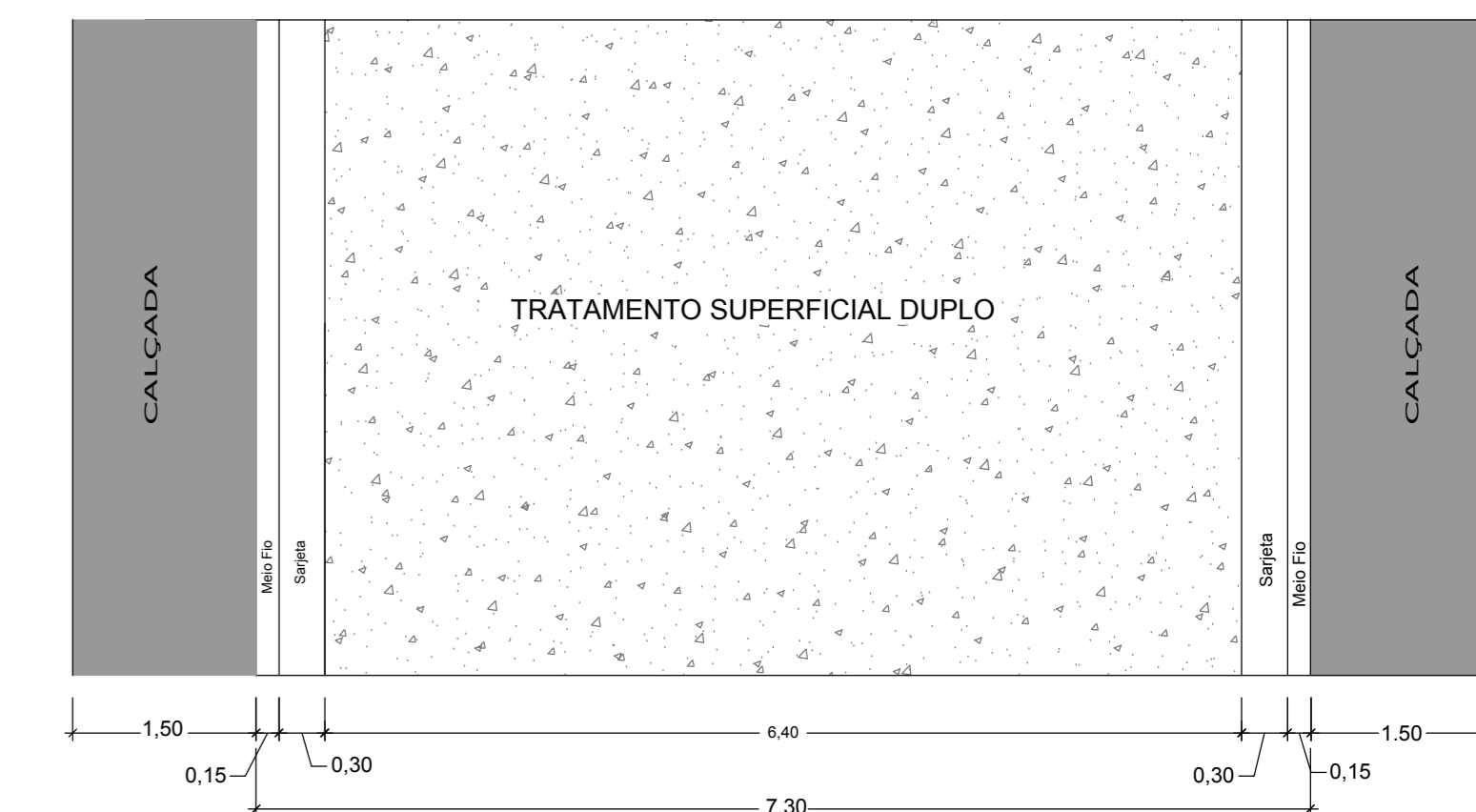
DETALHE DE VIAS
