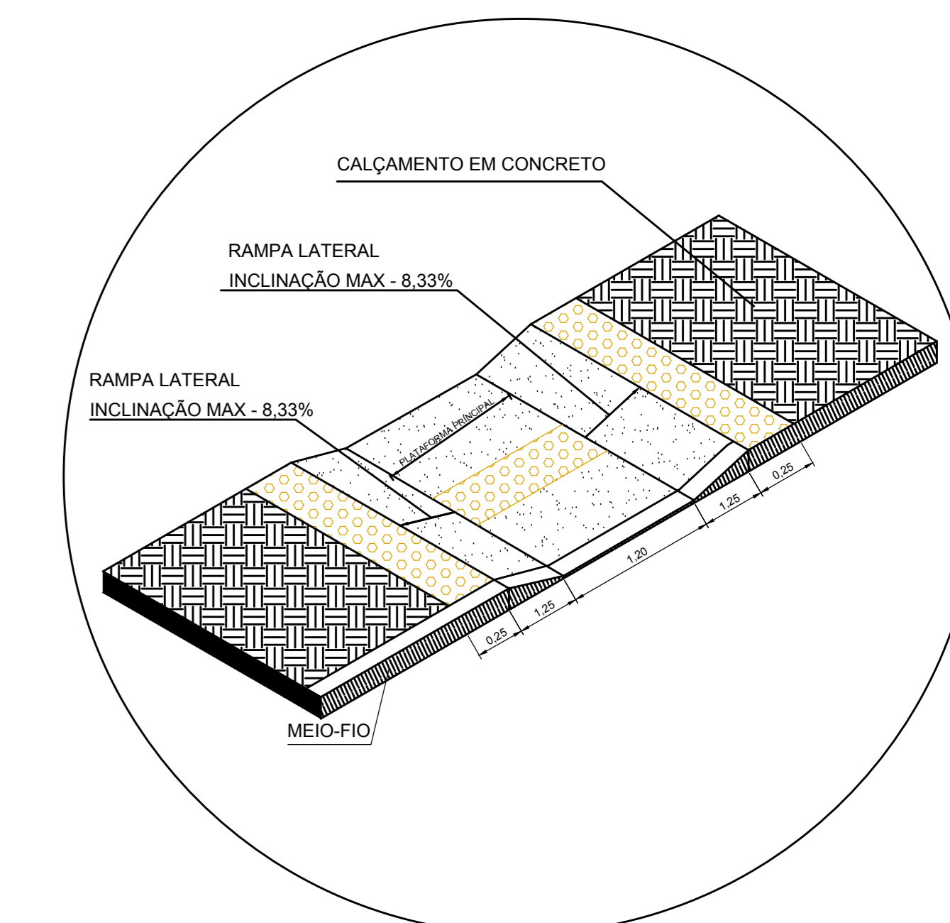
DETALHE DE RAMPA DE ACESSIBILIDADE
