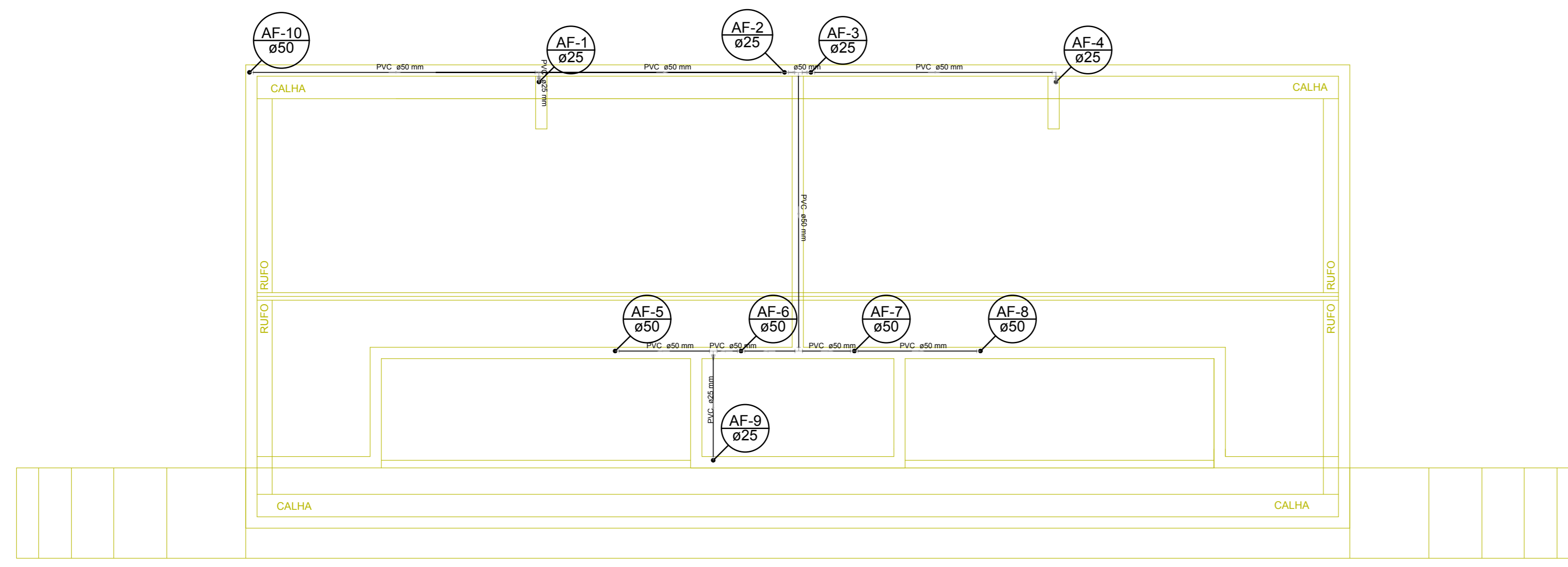
Planta de água fria da cobertura escala 1:50
